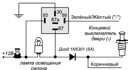
ЦЕПЬ ВНУТРИСАЛОННОГО ОСВЕЩЕНИЯ ОТРИЦАТЕЛЬНОЙ ПОЛЯРНОСТИ
