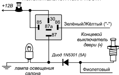
ЦЕПЬ ВНУТРИСАЛОННОГО ОСВЕЩЕНИЯ ПОЛОЖИТЕЛЬНОЙ ПОЛЯРНОСТИ
